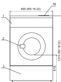
ПРЕДЕН RS 18 22
