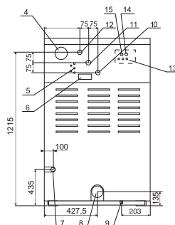
ЗАДЕН RS 18 22
