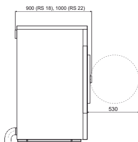
СТРАНА RS 18 22
